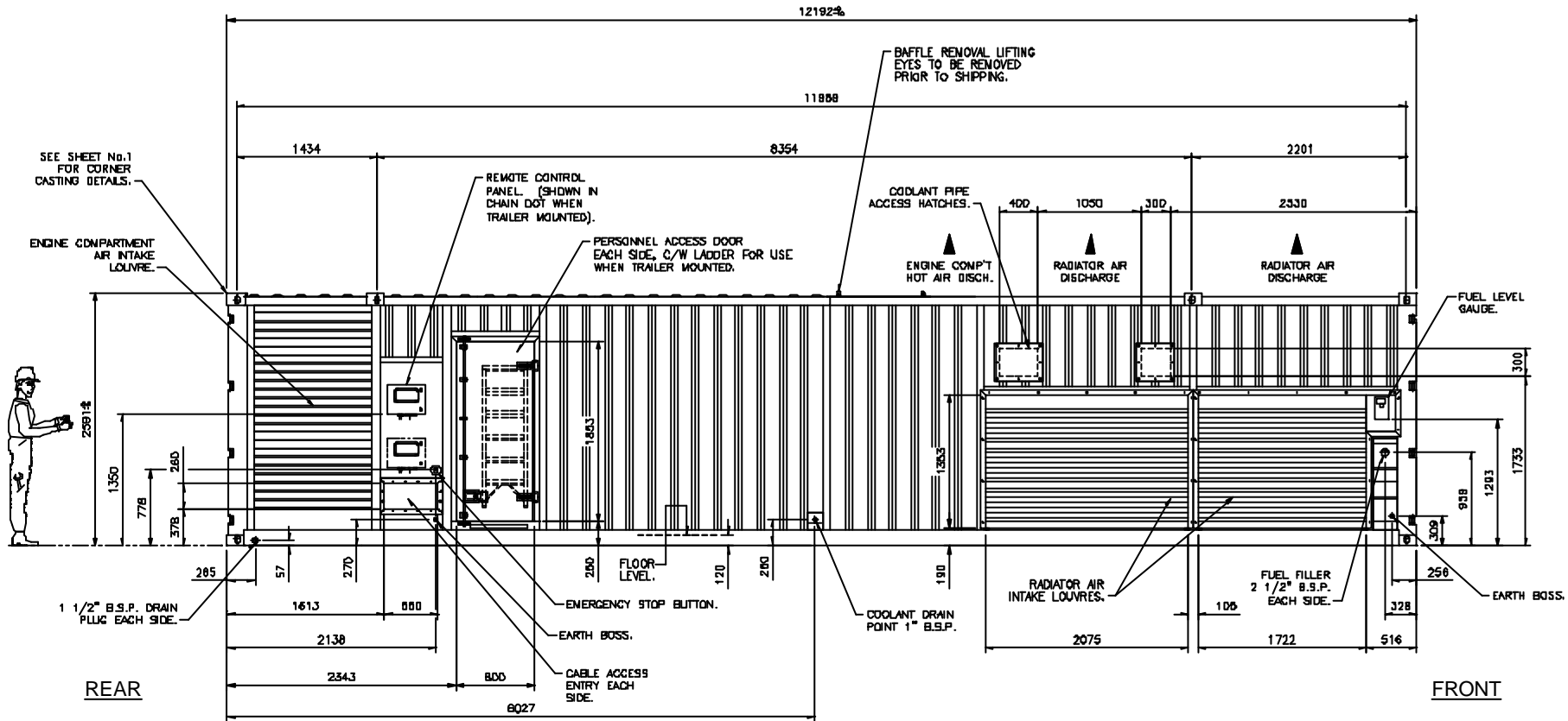
R.H.S. ELEVATION
